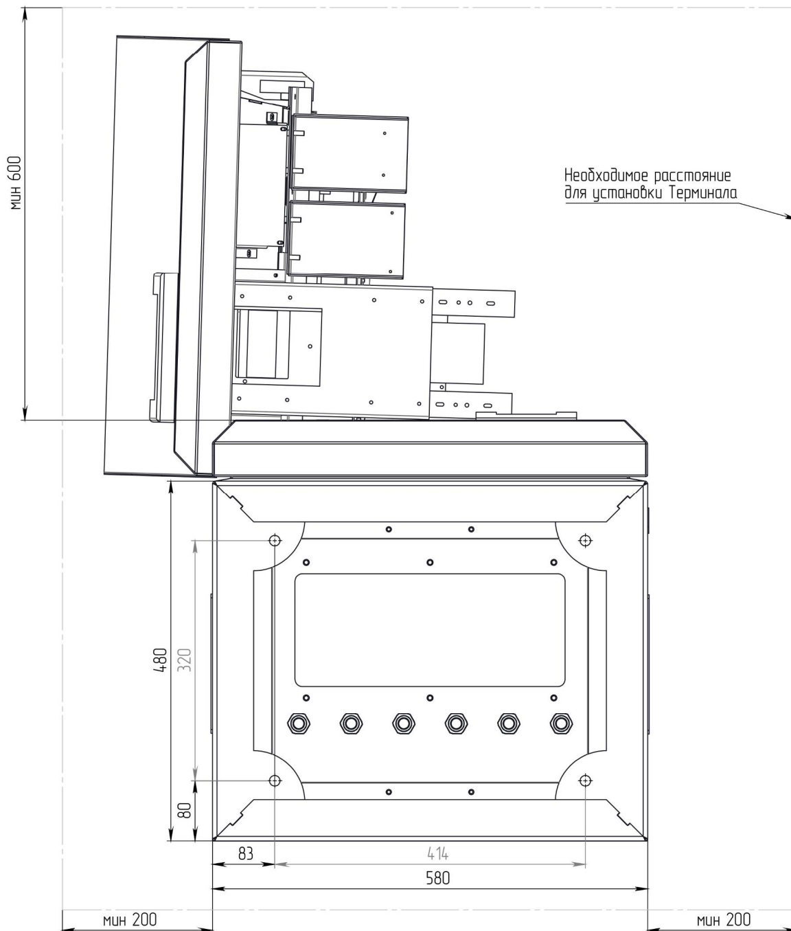
Установочные размеры
