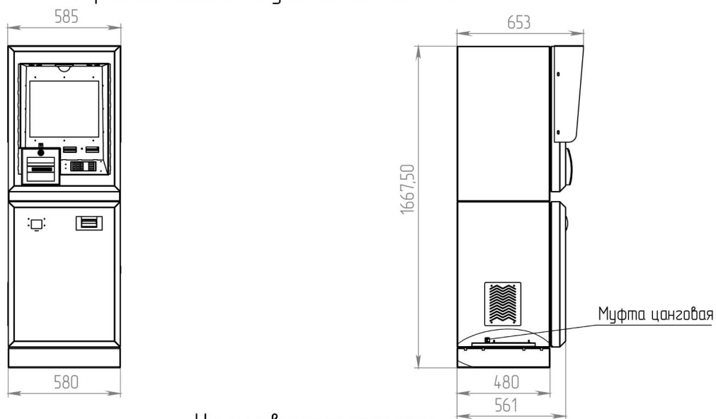
Установочные размеры
