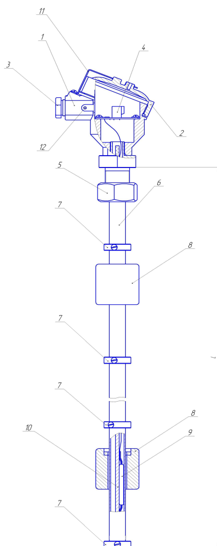
Рис. 2. Внешний вид датчика
